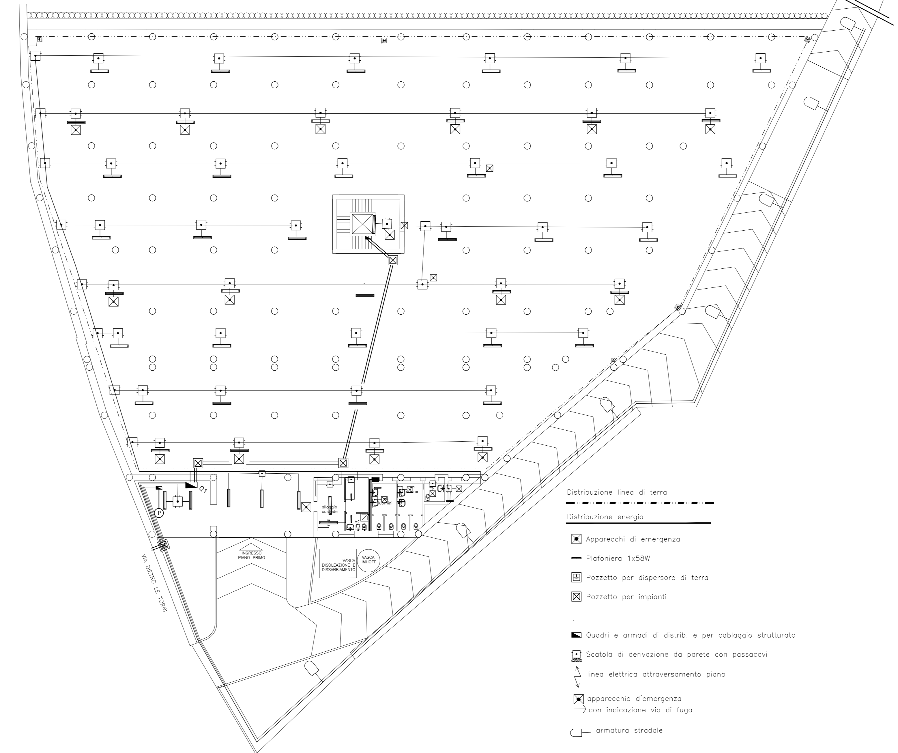
PIANTA STATO DI FATTO _scala 1/200 PIANO TERRA (PRIMO LIVELLO)
