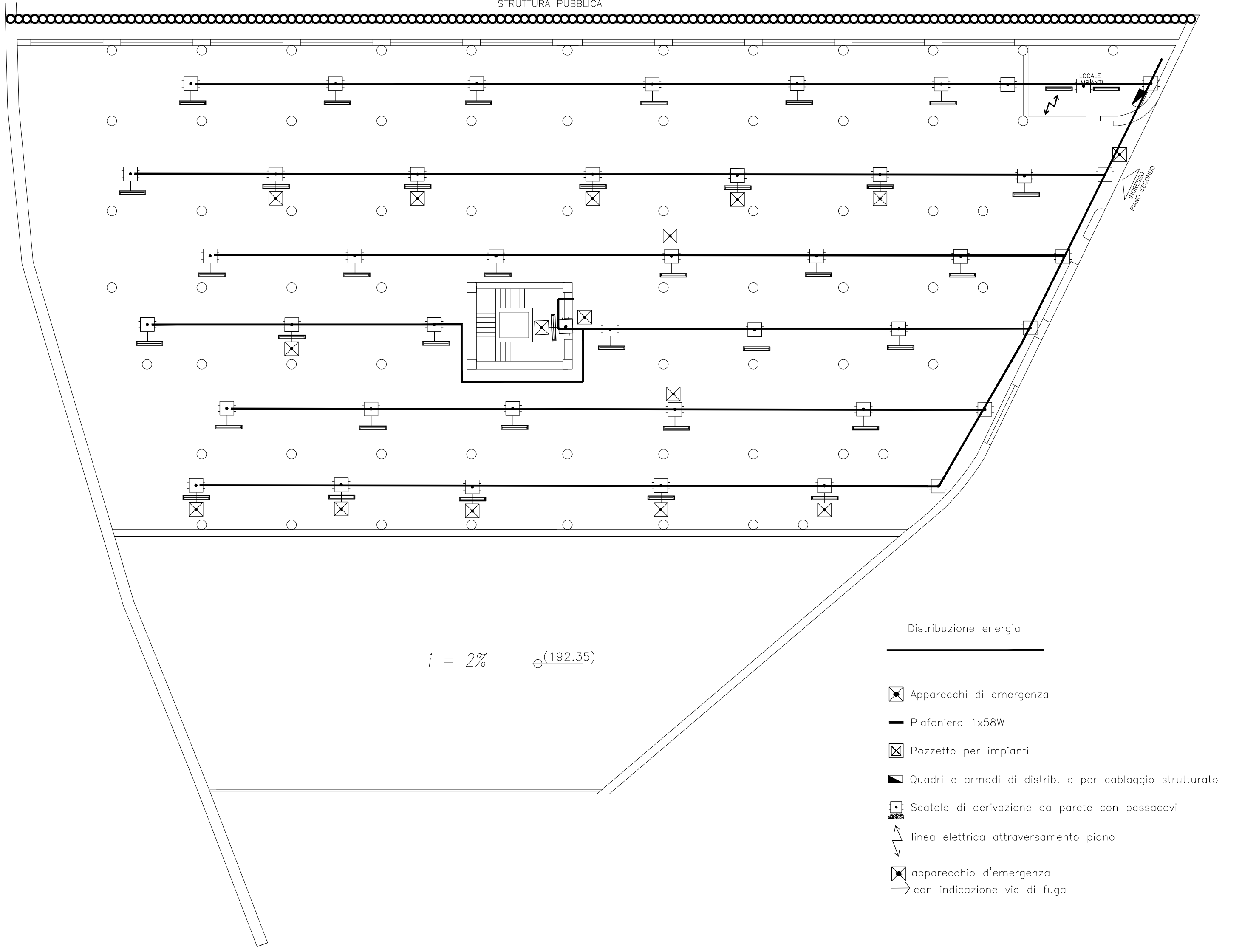
PIANTA STATO DI FATTO _ scala 1/200 PIANO PRIMO (SECONDO LIVELLO)
