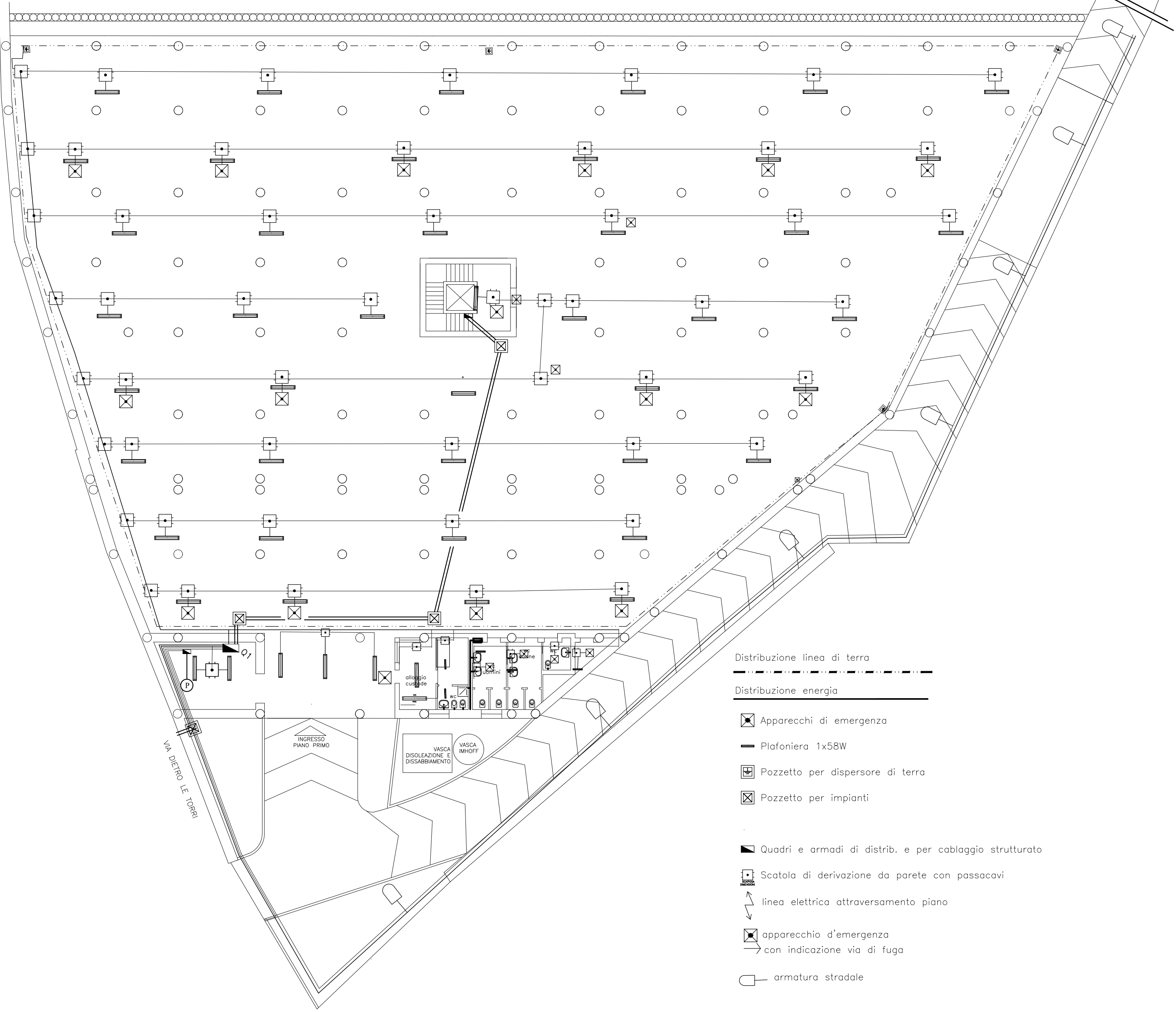
PIANTA STATO DI FATTO _ scala 1/200 PIANO TERRA (PRIMO LIVELLO)
